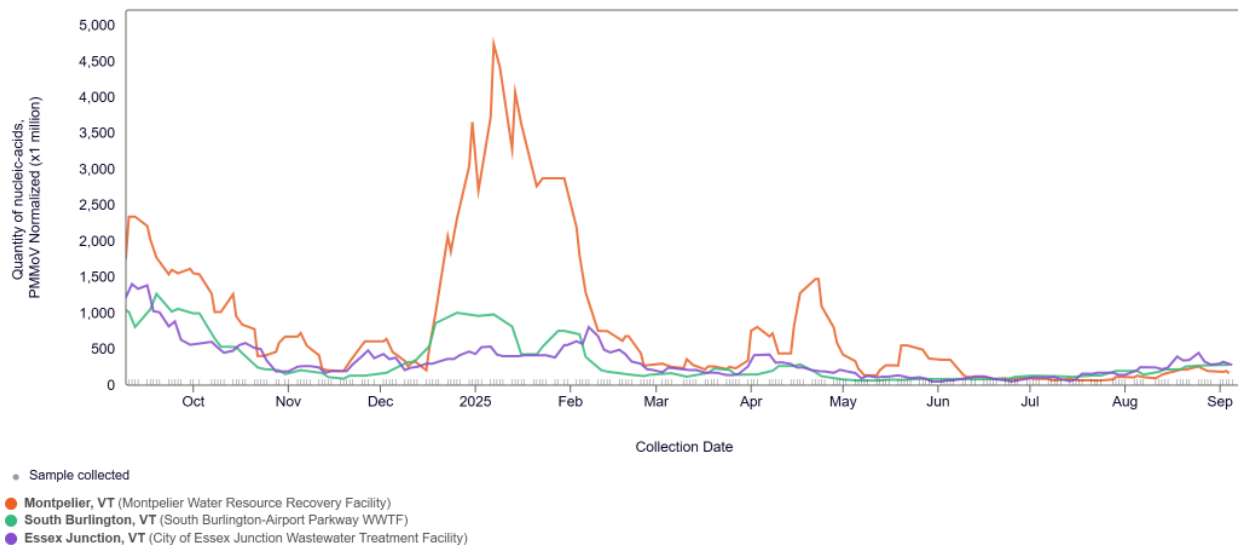
SARS-CoV-2, Vermont
