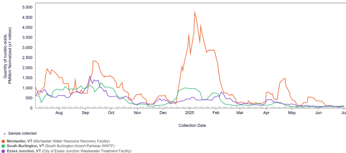
SARS-CoV-2, Vermont
