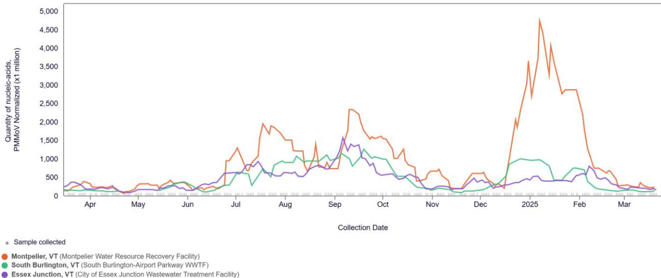
SARS-CoV-2, Vermont
